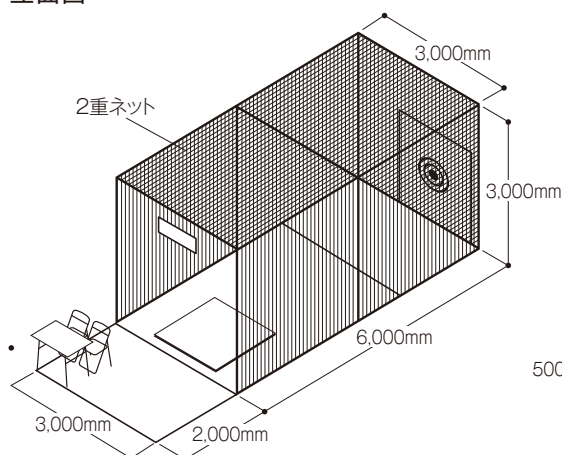
立面図
