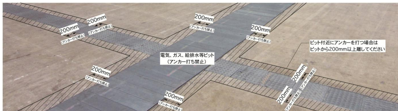
図1 床面アンカー施工不可エリアの説明図
