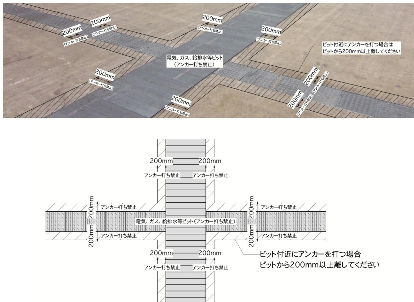
図1 床面アンカー施工不可エリアの説明図
