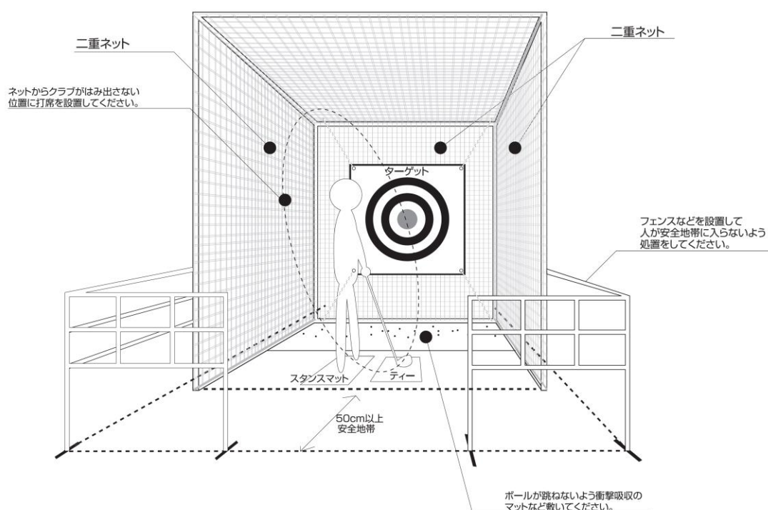
図2 2重ネット規定
