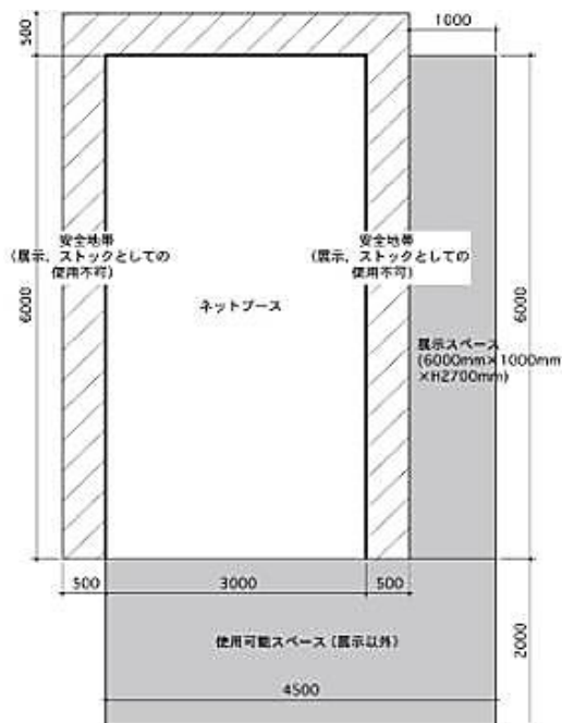
* 平面図
